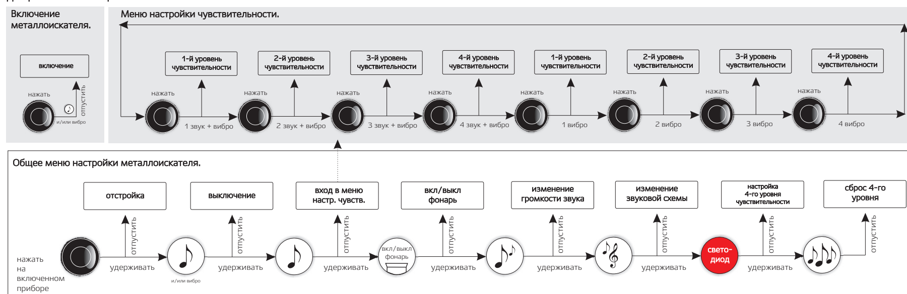
Диаграмма меню настроек металлоискателя
